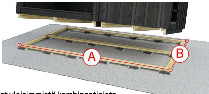
Perustusten mitat yleisimmistä kombinaatioista
