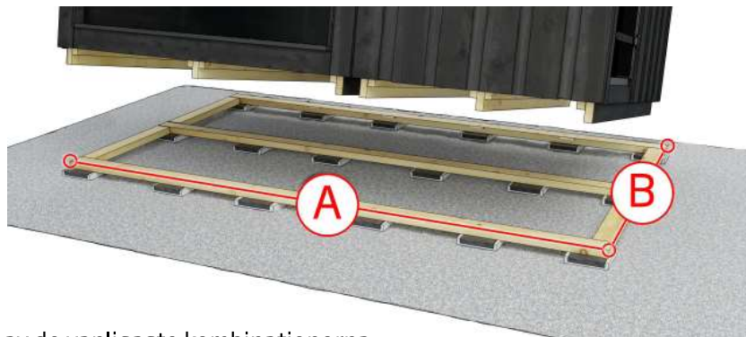
Mått på fundament av de vanligaste kombinationerna
