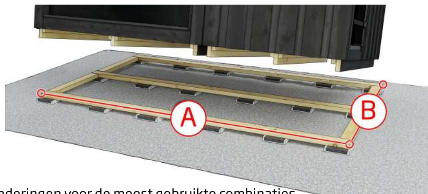
Afmetingen van funderingen voor de meest gebruikte combinaties
