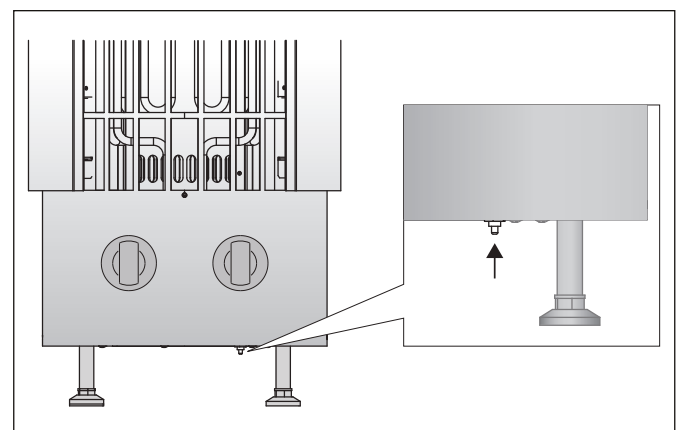
Figure 8. Réinitialiser les boutons pour les sécurités surchauffe.
