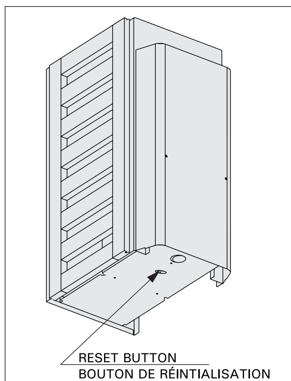
Figure 3. Place of the reset button Figure 3. Emplacement du bouton de réinitialisation
