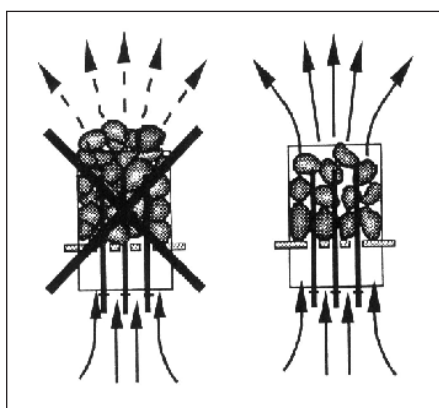
Figure 1. Piling of the sauna rocks Figure 1. Mise en place des pierres du poêle
