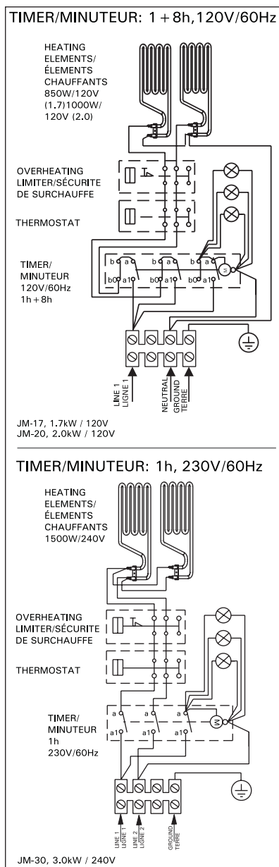
Figure 10. Connexions électriques des poêles
