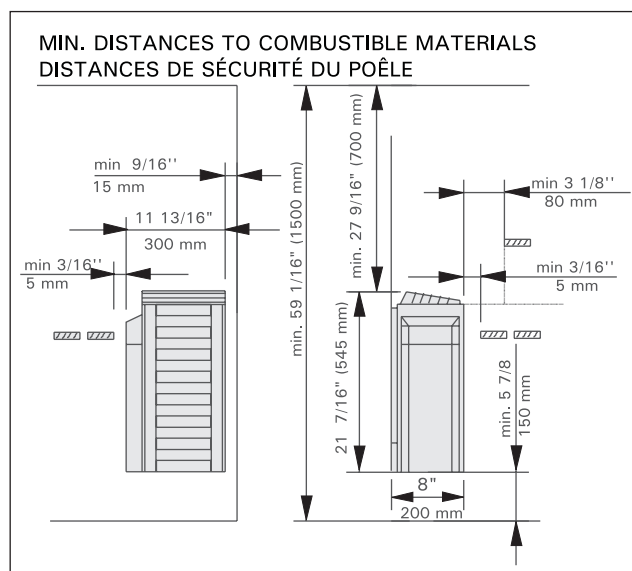
Figure 5. Min. distances to combustible materials Figure 5. Distances de sécurité du poêle
